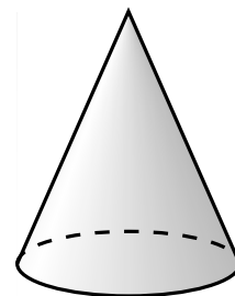
cone
